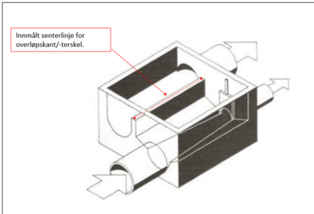
Figur 12: Innmåling på overløpskant.
