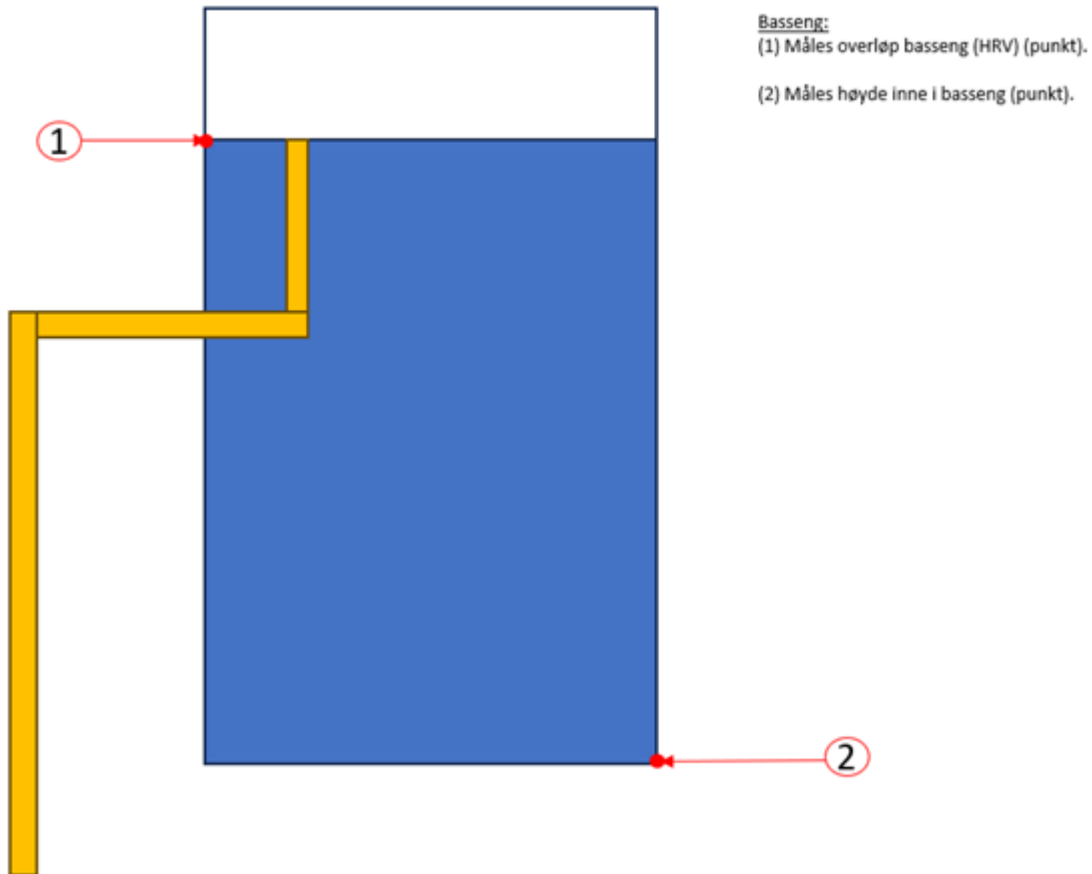
Figur 15: Innmåling av høydebasseng.
