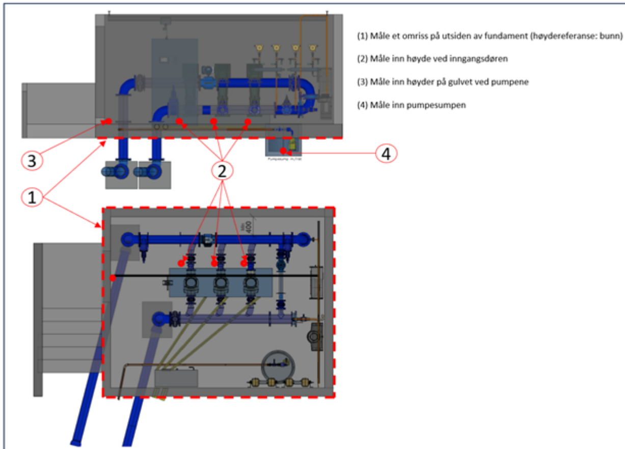
Figur 14: Innmåling av vannpumpestasjon.
