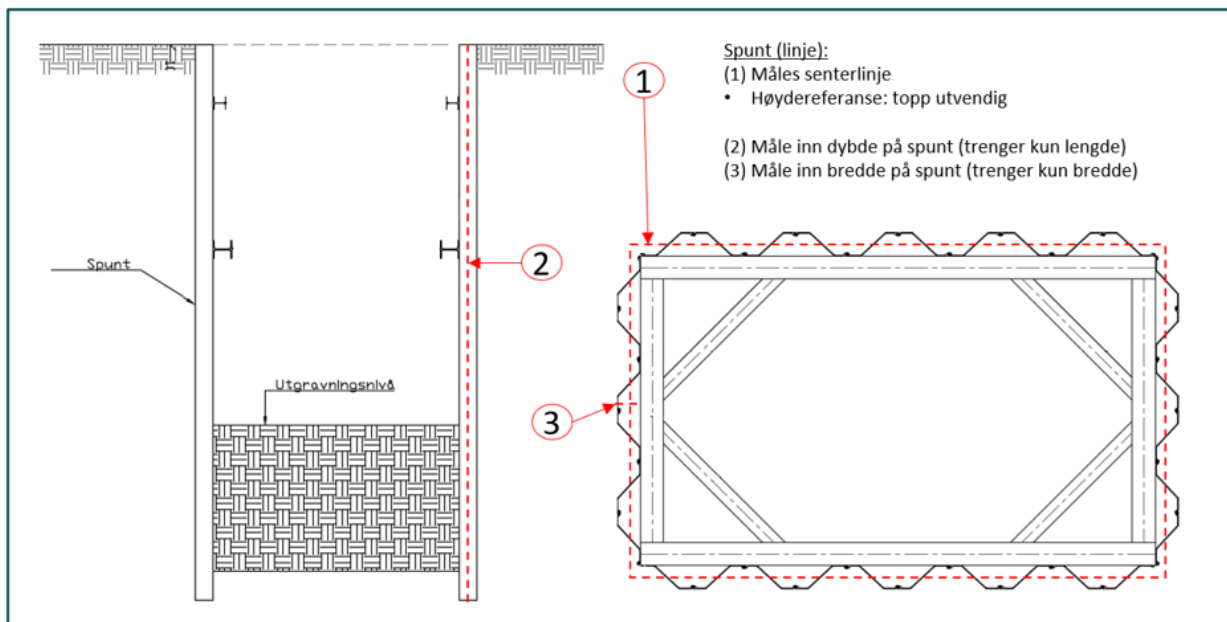
Figur 16: Innmåling av spunt.
