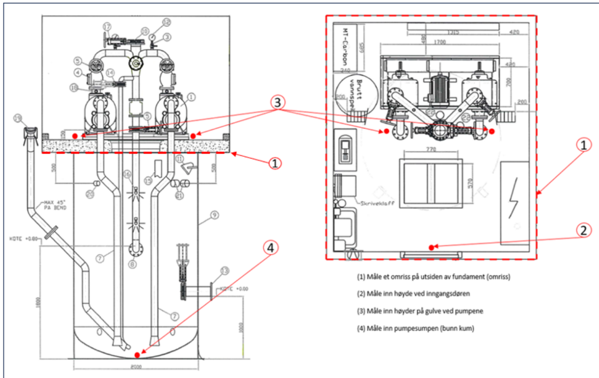
Figur 13: Innmåling av avløpsumpe.
