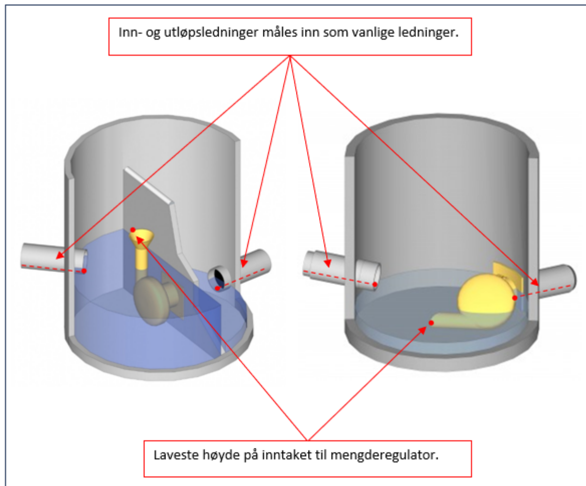
Figur 11: Eksempel på utløpskum med mengderegulator med innmålingspunkter.
