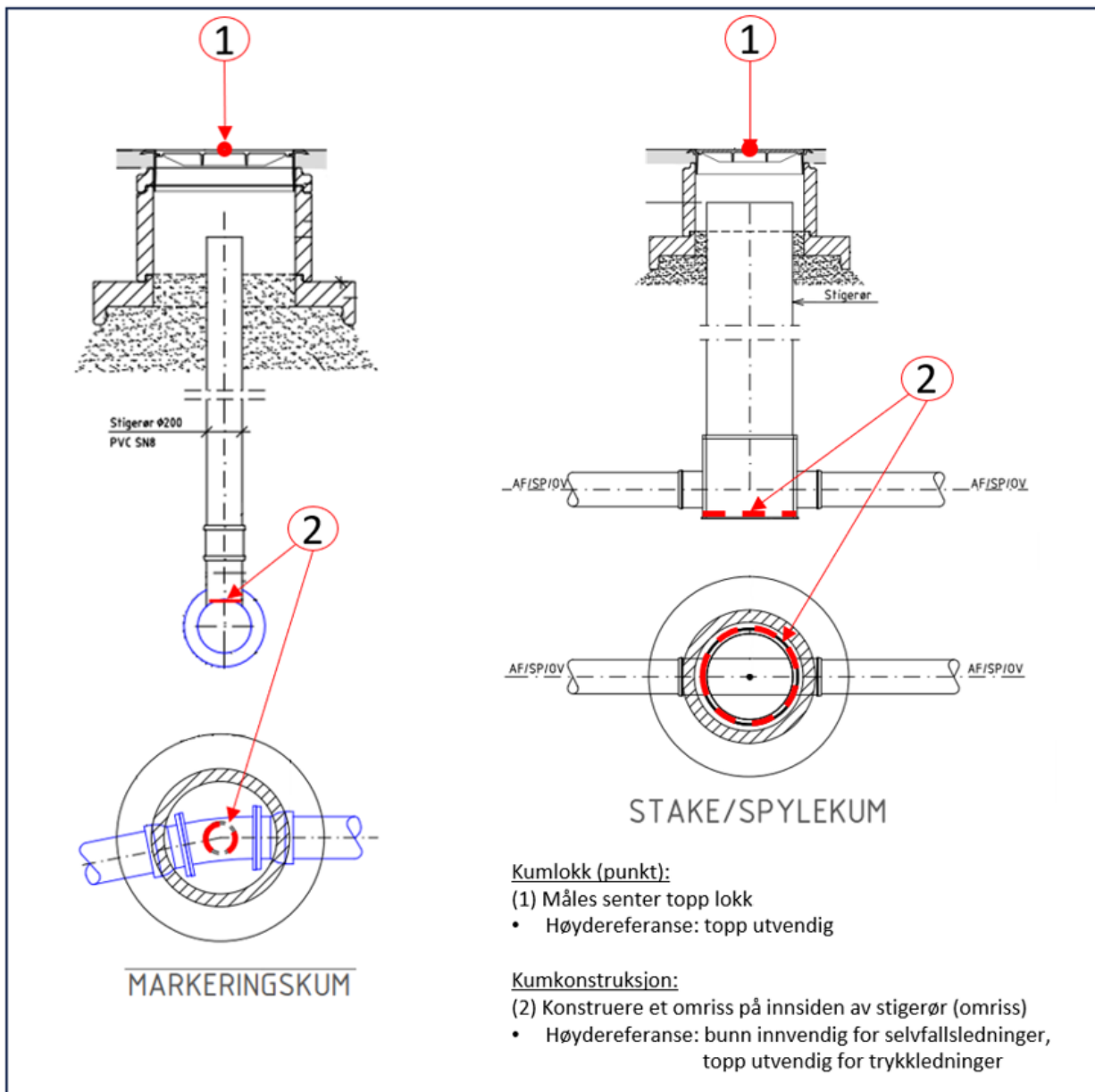
Figur 9: Innmåling av markerings/stake/spylekum.
