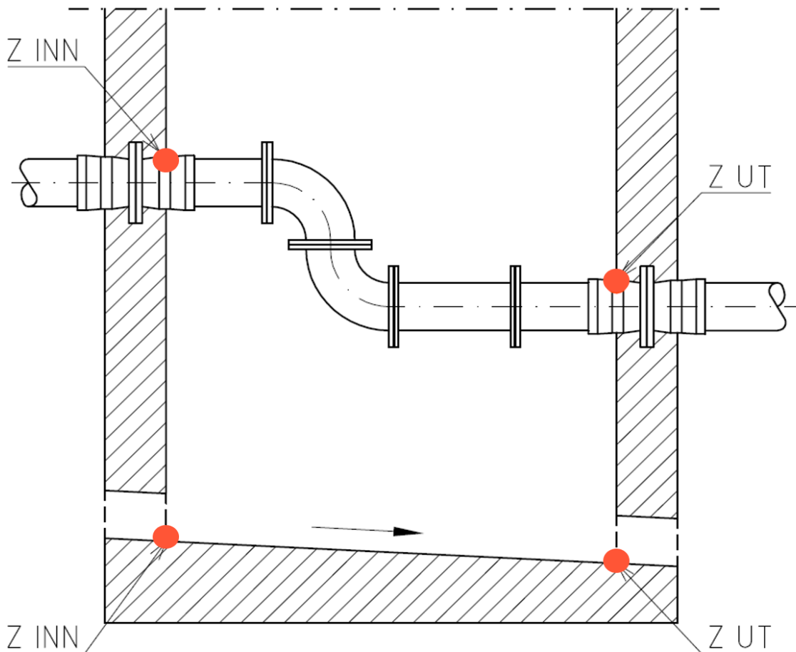
Figur 17: Innmåling av høyder på ledninger i kum.
