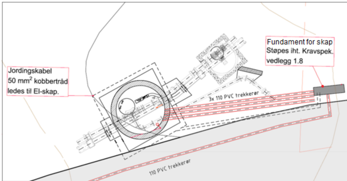
Figur 21: Elektroanlegg.
