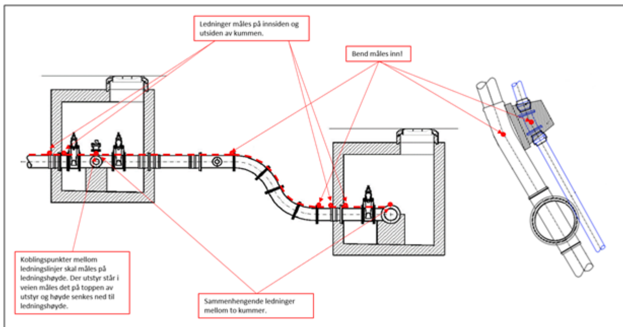
Figur 3: Innmåling av ledning mellom kummer og innmåling av bend.
