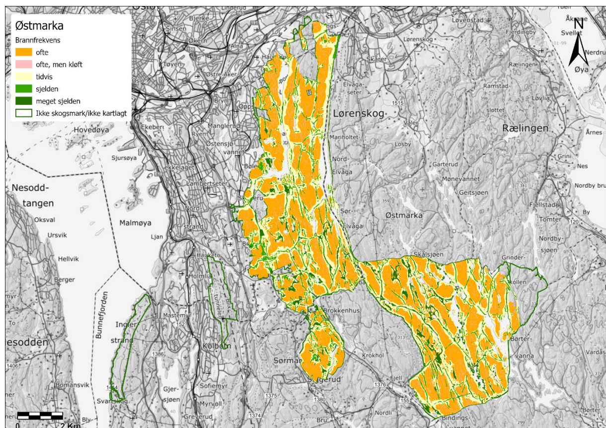
Figur 19. Landskapsanalysen for Østmarka baseres på brannfrekvens, dvs. at brann ville ha vært den viktigste forstyrrelsesfaktoren i en naturskogstilstand.
