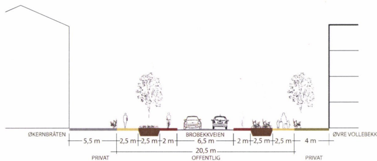
Brobekkveien - tverrsnitt Øvre Vollebekk 1:400 (AA)
