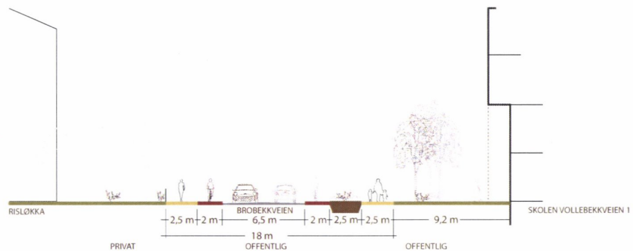
Brobekkveien - tverrsnitt ved skolen 1:400 (BB)
