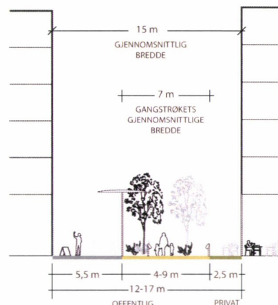
Gangstrøket - tverrsnitt Nedre Vollebekk 1:400 (BB)
