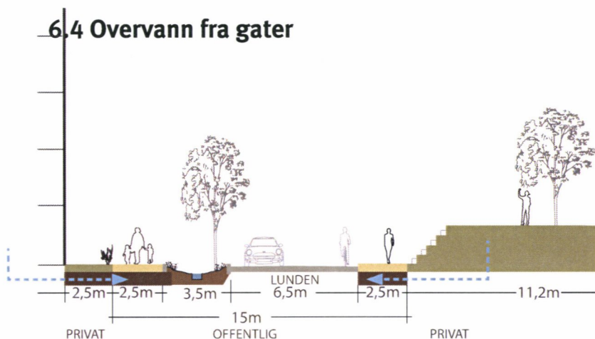
Lunden med bekkeåpning - tverrsnitt Øvre Vollebekk 1:300
