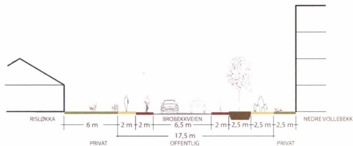
Brobekkveien - tverrsnitt Nedre Vollebekk 1:400 (CC)
