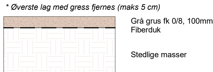
Prinsipp oppbygging komprimert subbus, 1:20
