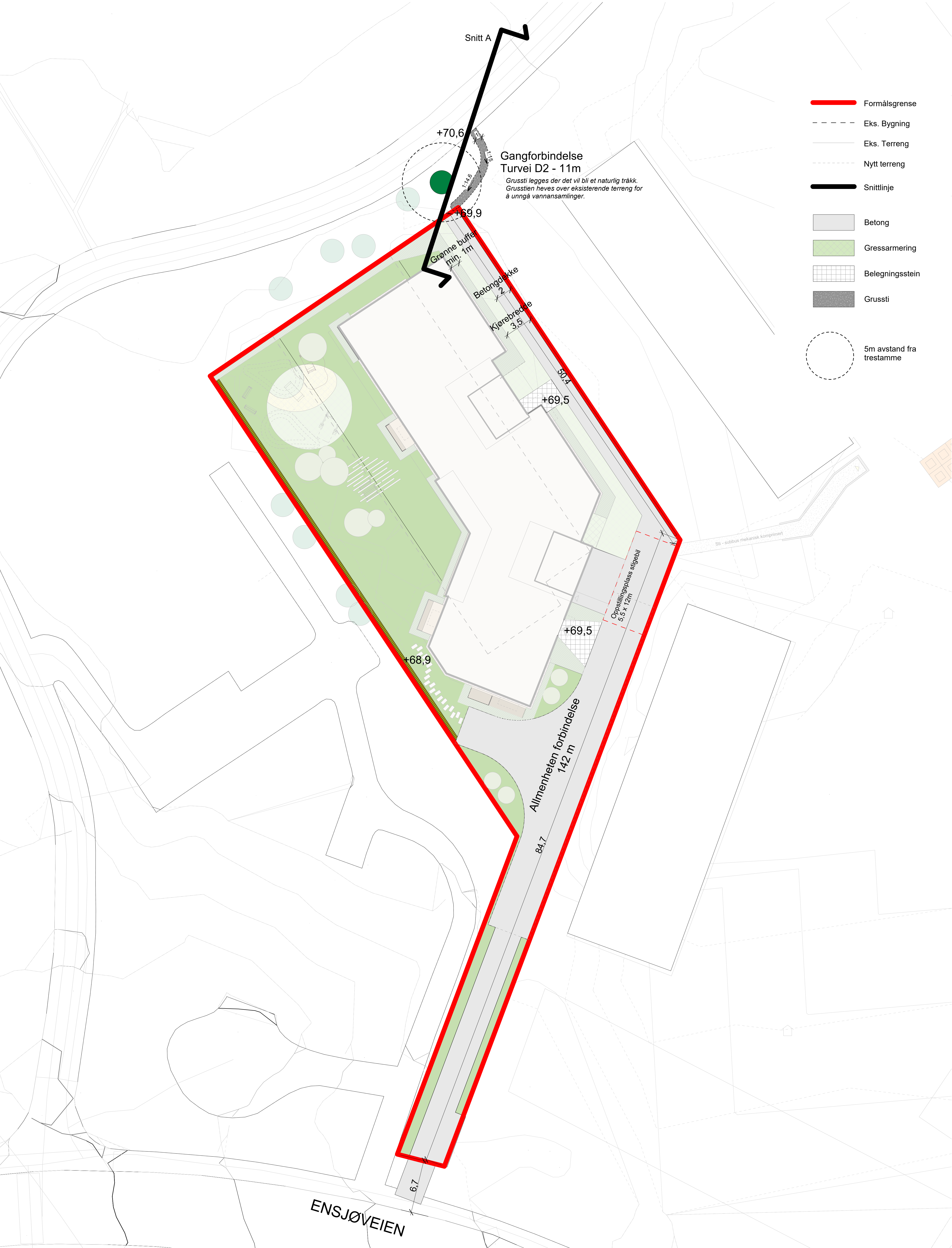
Oversikt Gangforbindelse med turvei D2 - 1:200
