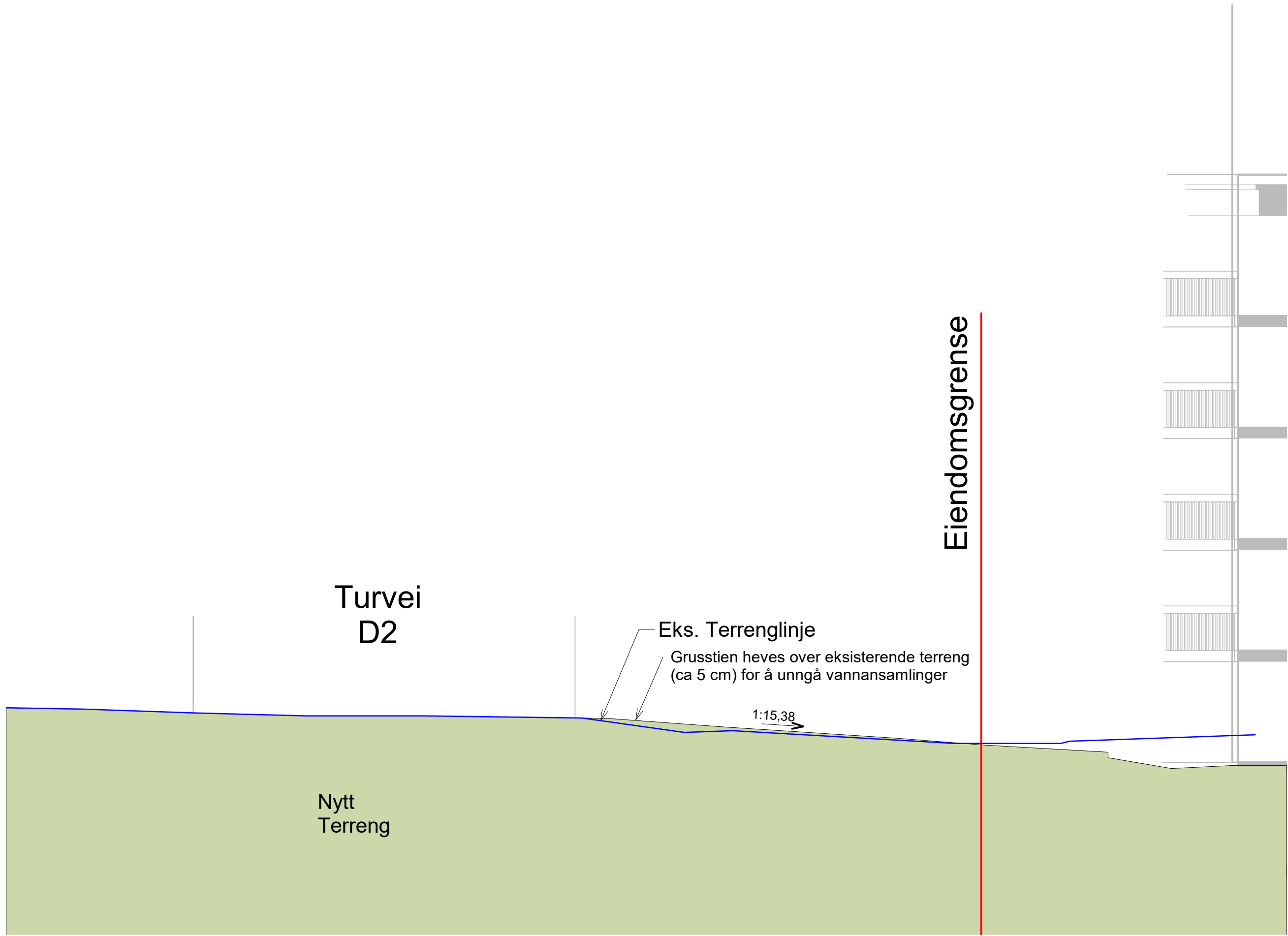
Snitt A - 1:100
