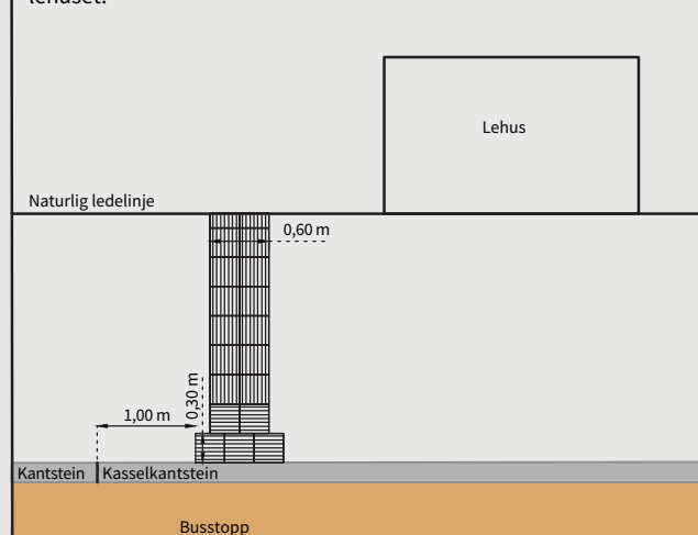
Ledelinje på busstopp med forskjøvet lehus. Retningsindikator avsluttes mot naturlig ledelinje som leder til lehuset.
