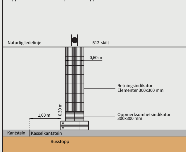
Oppmerksomhetsfelt på busstopp med kun 512 skilt.
