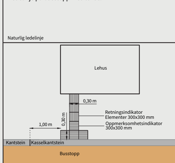
Ledelinje på busstopp med lehus.
