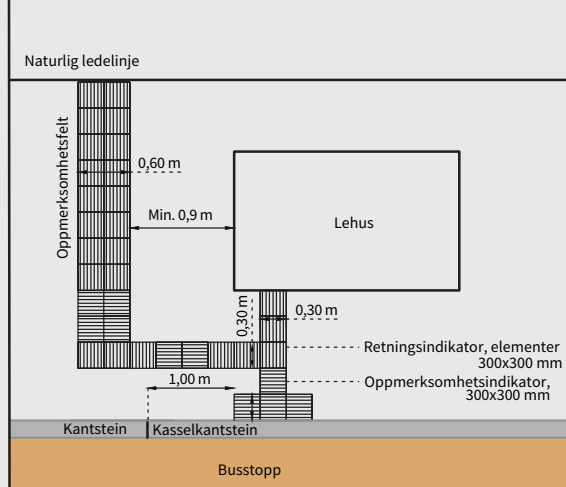
Ledelinje på busstopp med lehus som ligger ut fra veggen. Her bør oppmerksomhetsfelt gå helt til veggen.
