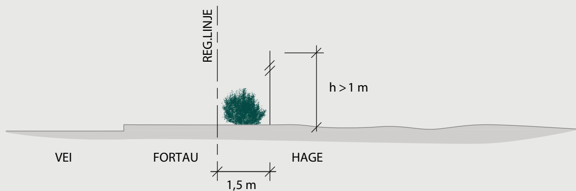
Fig. 2: Plassering av høyt tett gjerde / skjerm i veiprofilet
