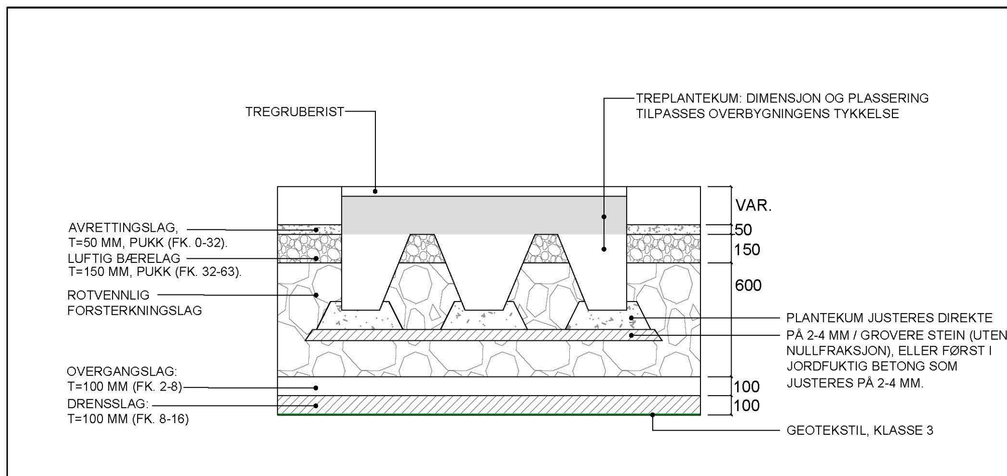
PRINSIPPSNITT TREPLANTEKUM, TYPE A
