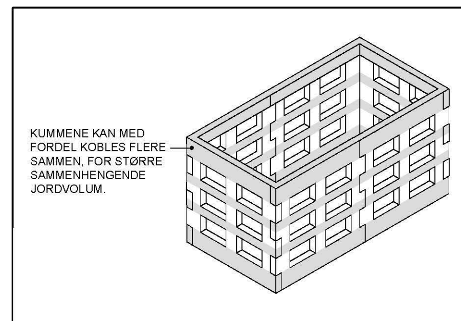
SAMMENKOBLING TREPLANTEKUMMER, TYPE C
