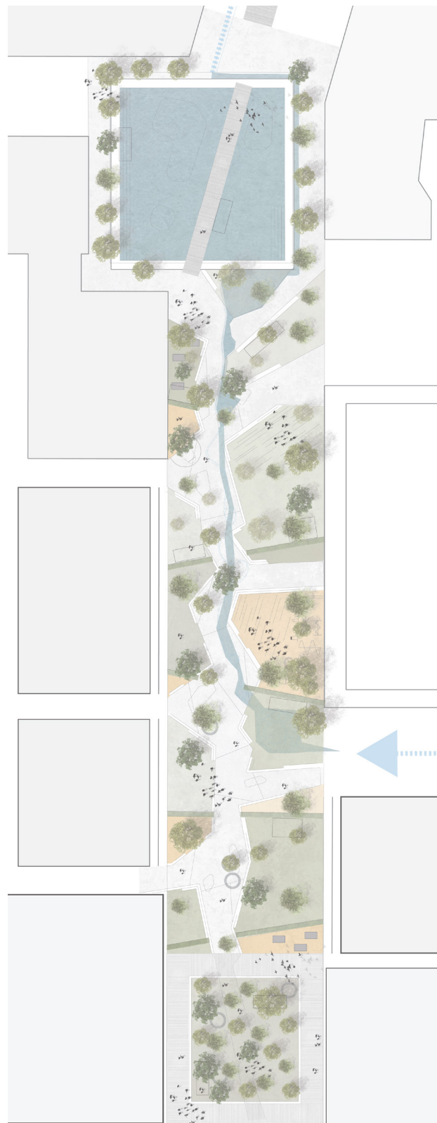
Gjenåpning av bekken, presentert på alnainvolverer.no
