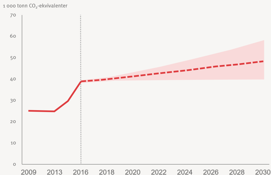
Figur 4: Utslippsstatus for sjøfart i Oslo kommune fram til 2016, og hvordan utslippene kan utvikle seg fram mot 2030. Skravert område indikerer usikkerestimatet. Figuren er basert på data fra Miljødirektoratet og CICERO.
