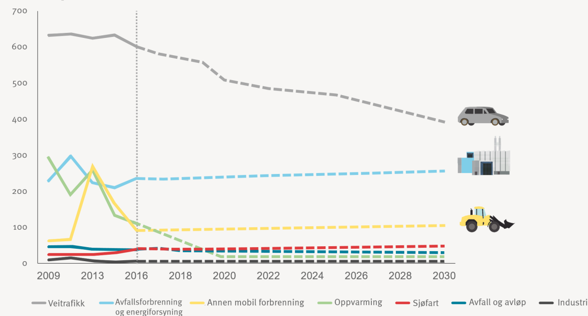
Figur 1: Øverst: Utslipp av klimagasser fra alle sektorer fra 2009 til 2016 (hel linje). Fra 2016 er figuren en framskriving for Oslos klimagassutslipp fram mot 2030 uten nye tiltak (stiplet linje). Skravert område viser utsikkerhet. Nederst: Utslipp av klimagasser fordelt på sektorer fra 2009 til 2016 (hel linje). Fra 2016 er figuren en framskriving for Oslos klimagassutslipp fram mot 2030 uten nye tiltak (stiplete linjer). Skravert område viser utsikkerhet. Figurene er basert på data fra Miljødirektoratet og CICERO.
