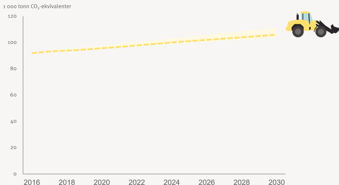
Figur 5: Hvordan utslippene kan utvikle seg fram mot 2030 i sektoren bygge- og anleggsvirksomhet. Skravert område viser utsikkerhetsestimatet. Figuren er basert på data fra CICERO.
