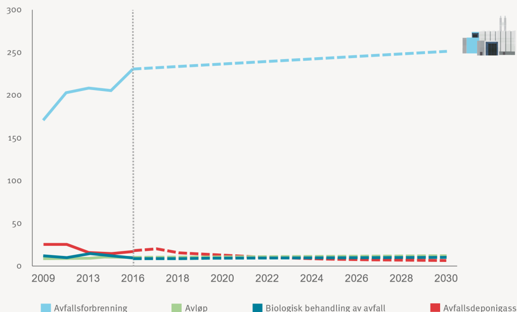
Figur 6: Utslipp av klimagasser innen avfall og avløp fram til 2016, og hvordan utslippene kan utvikle seg fram mot 2030. Figuren er basert på data fra Miljødirektoratet og CICERO.
