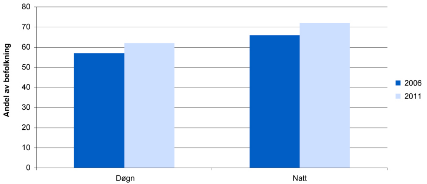
Figur 10.3 Andel av befolkning som er utsatt for støy fra vei og bane høyere enn 55 dB i gjennomsnitt i døgnet og 45 dB i gjennomsnitt om natten
