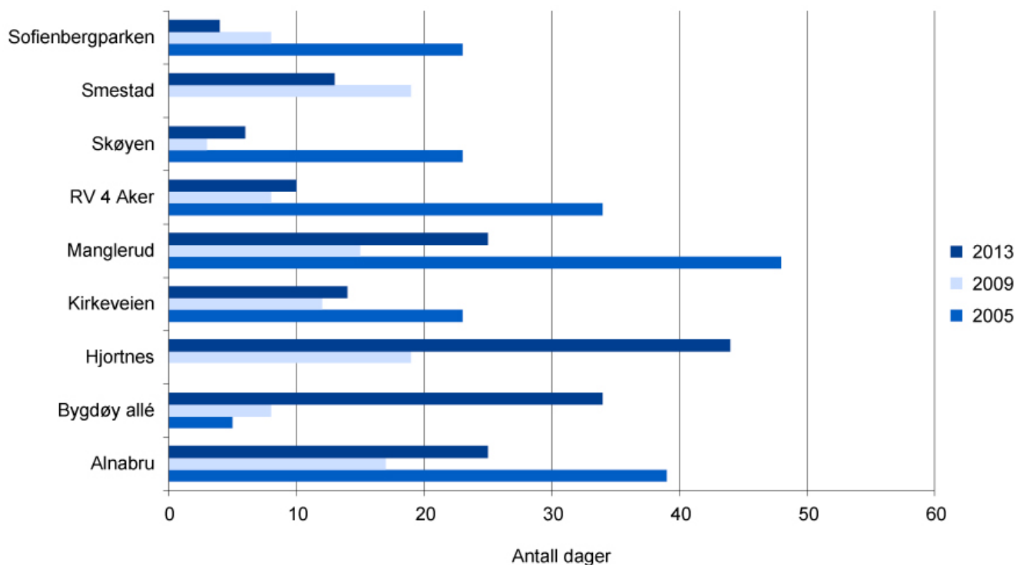
Figur 10.2 Antall dager i året hvor konsentrasjonen av svevestøv er over anbefalt grenseverdi
