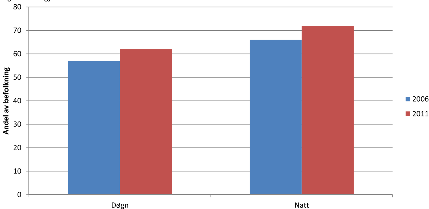
Figur 10.3 Andel av befolkning som er utsatt for støy fra vei og bane høyere enn 55 dB i gjennomsnitt i døgnet og 45 dB i gjennomsnitt om natten
