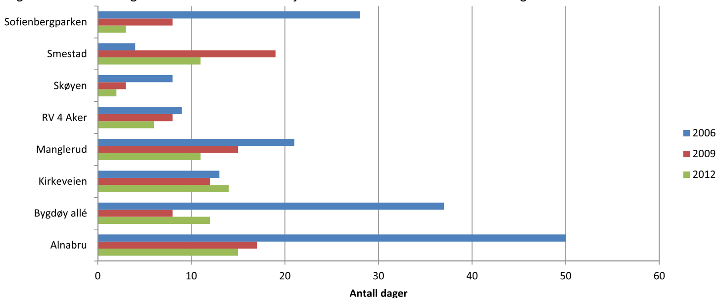
Figur 10.2 Antall dager i året hvor konsentrasjonen av svevestøv er over anbefalt grenseverdi
