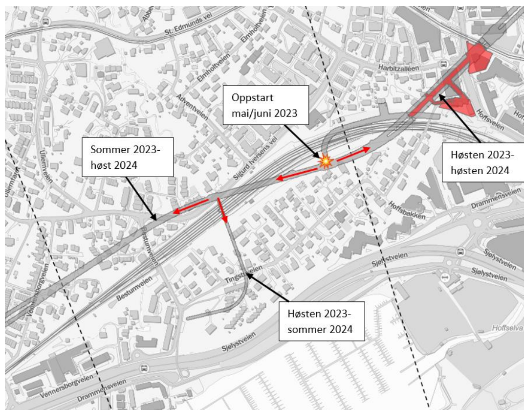
Figur 1: Oversikt over planlagt framdrift tunneldriving på strekningen Skøyen - Vækerø.
