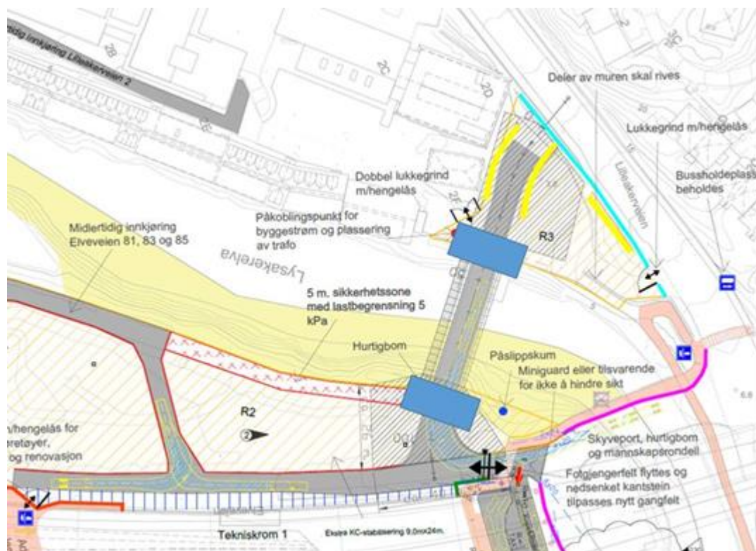
Figur 1: Gul linje markerer der spunten skal ned. Blått felt markerer boring av stålkjernepeler.
