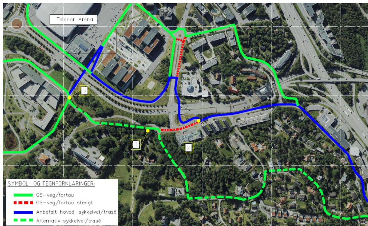
Figur 2: Overordnet plan for omleggingen av gang- og sykkeltrafikk i byggeperioden.
