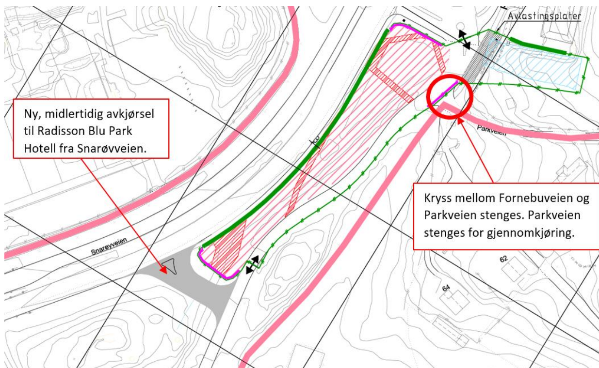
Figur 3: Utsnitt fra faseplan for bygging som viser anleggsområdets avgrensning samt ny, midlertidig avkjørsel til Radisson Blu Park Hotell fra Snarøyveien i grått nederst i figuren.
