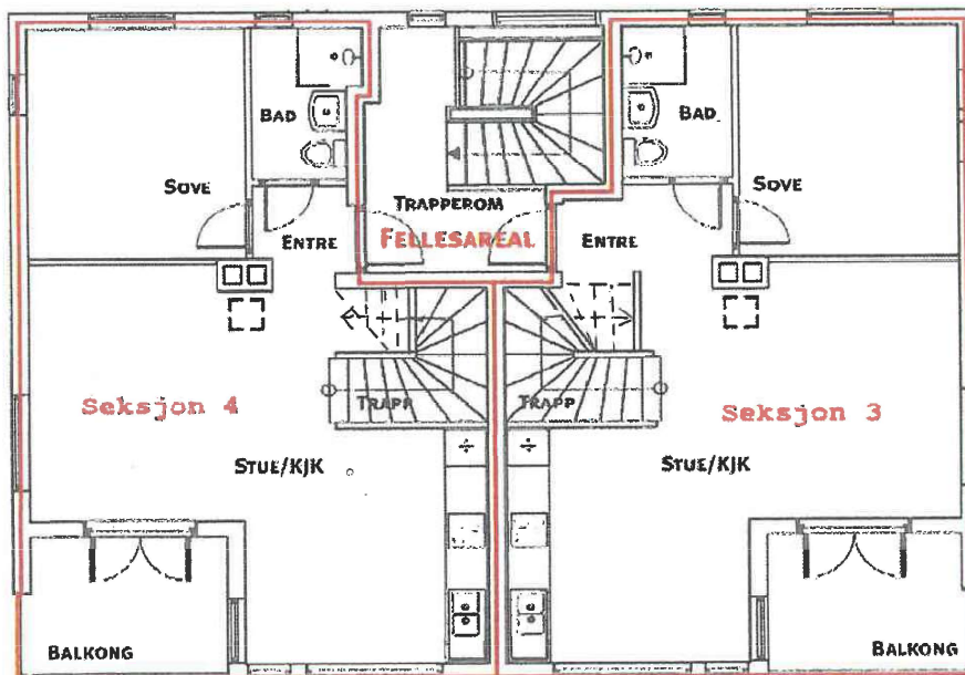
2. Etasje
