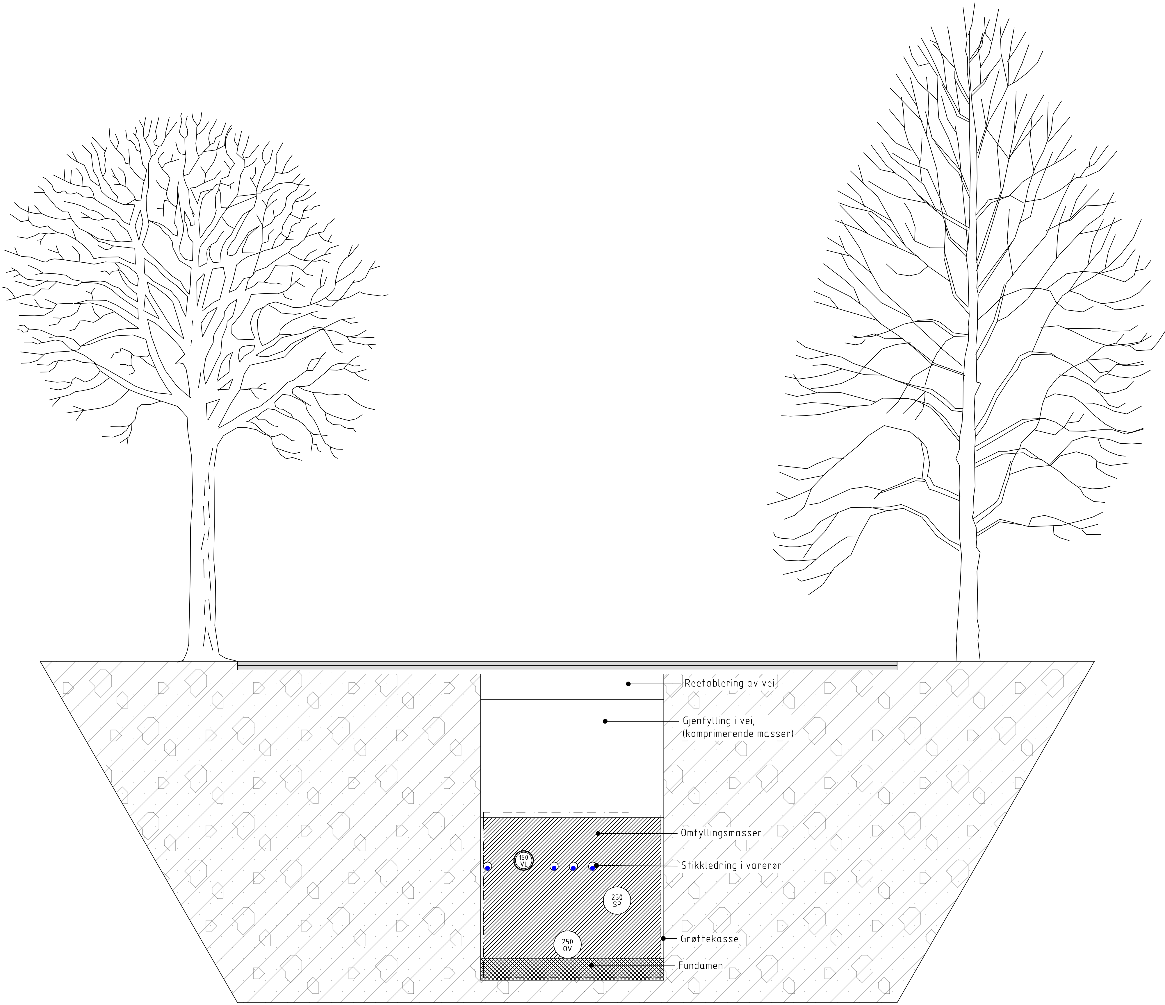
Grøftesnitt ledningstrase
