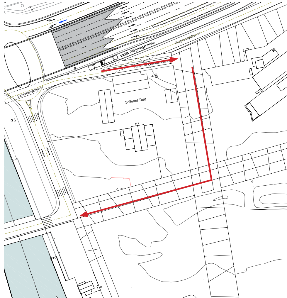
Atkomst til KLP og Frantzebråten fra i samme kryss som E18 legges på sørsiden av Sollerud gård.
