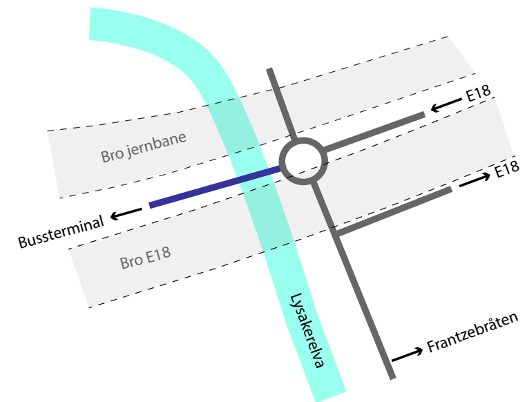
Alt K2A: Rundkjøring og lyskryss
