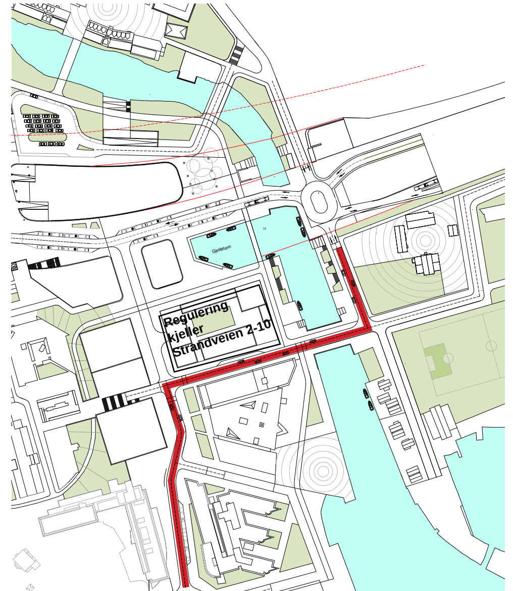
Figur 3. Regulering flyttet til kjeller i transformert Strandveien, Arealet under E18 kan da benyttes til andre formål.
