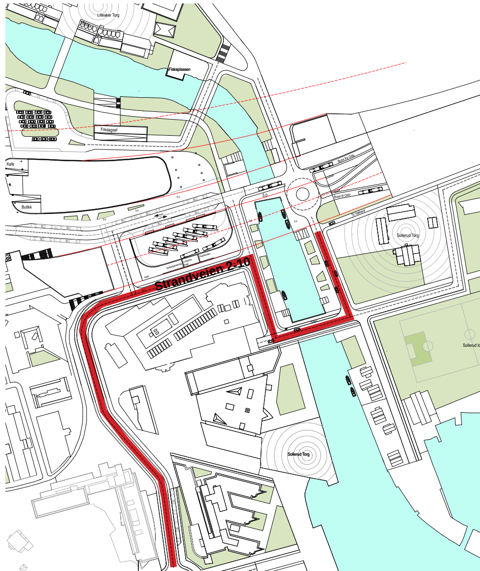
Figur 1. Bro flyttet mot sør. Strandveien 2-10 som i dag.
