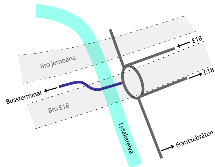
Alt K2B: Stor rundkjøring 1
