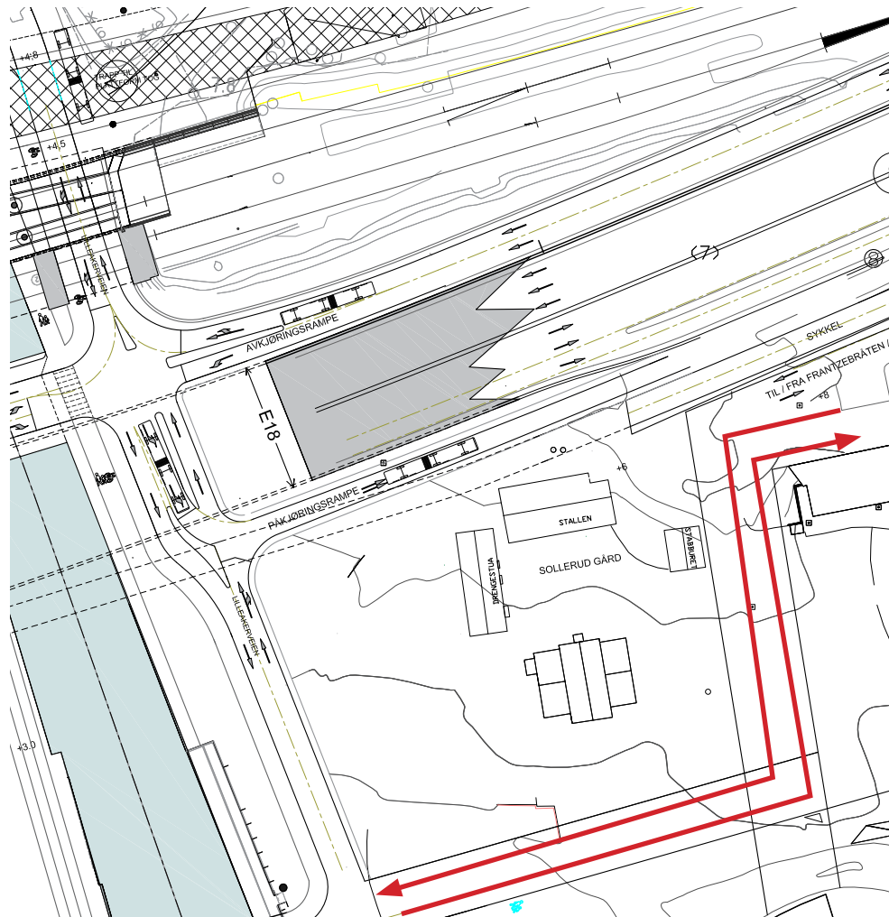
Atkomst til KLP og Frantzebråten legges på sørsiden av Sollerud gård og uavhengig av rampesystemet til E18.
