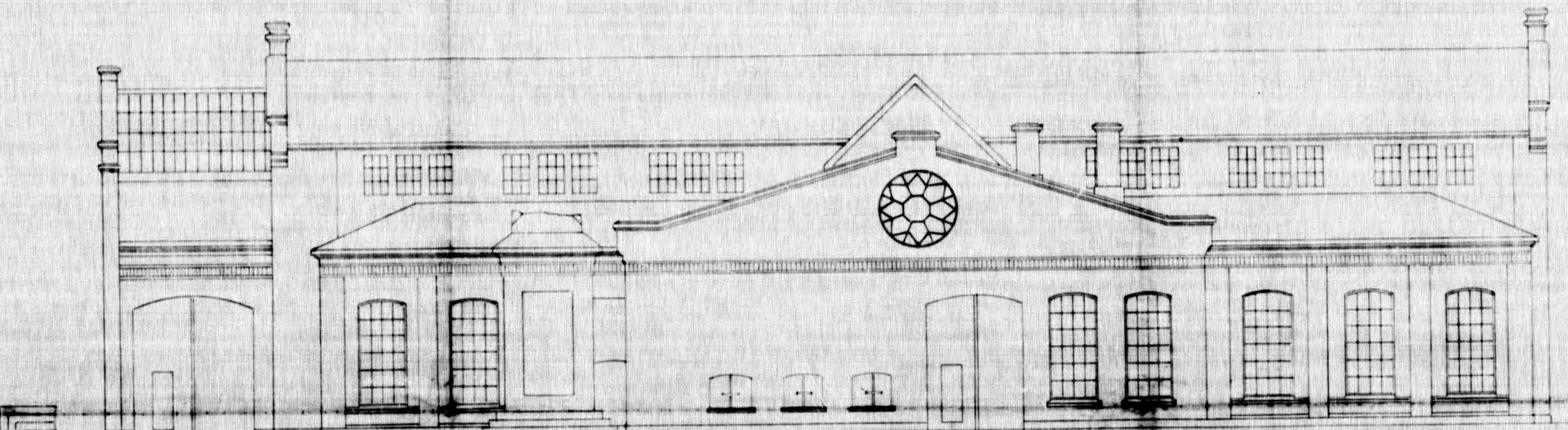
Façade mod N. O.
