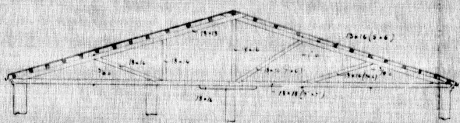
Tagetol over Maskinrum.
