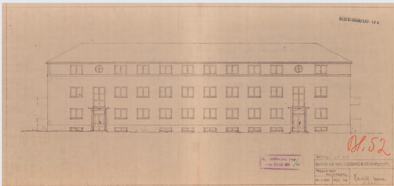
▼ Fasaden til Akersveien 28 , byggesakstegning. Oslo byarkiv Plan- og bygningsetaten, byggesaksarkiv 218/30
